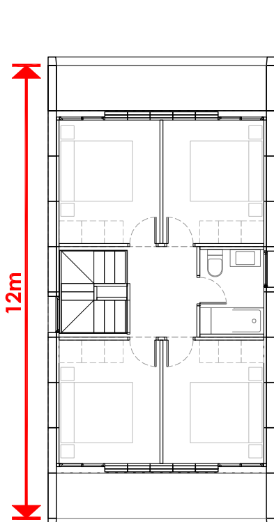
PLANTA PRIMERA
