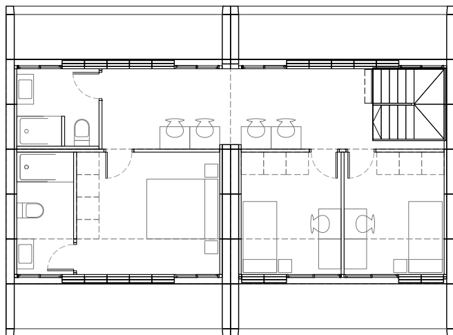
PLANTA PRIMERA
